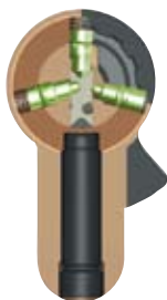
Устройство цилиндра
